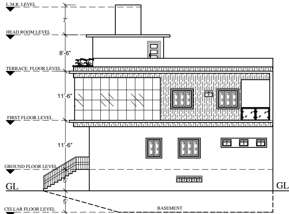
NW- ELEVATION
